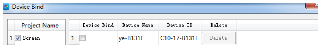
Fig. 4-1 Devise Bind
