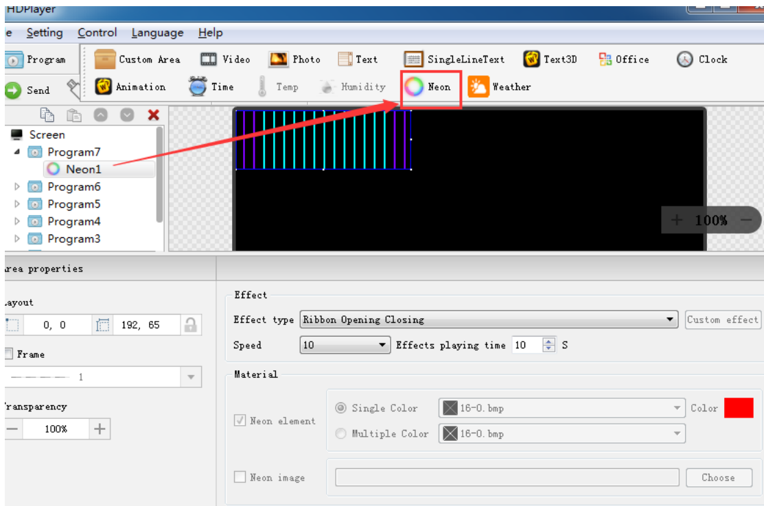
Fig. 7-33 Add Neon
